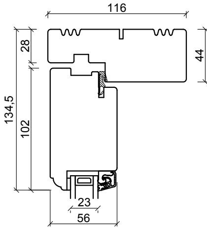
Toppkarm
