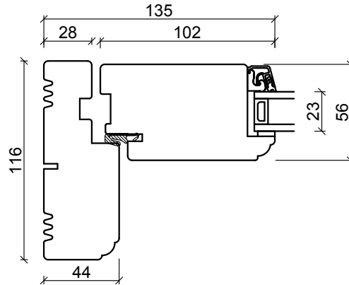
Sidokarm
