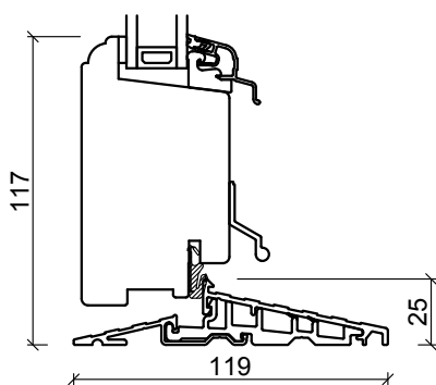
Bottenkarm (Alu-Tröskel:)
