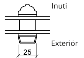
Spröjsar
