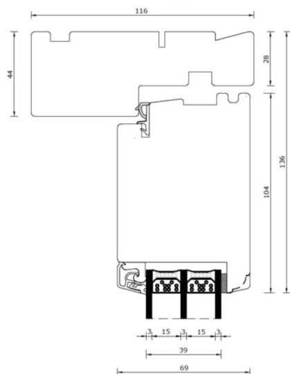
Hårdträ bottenkarm
