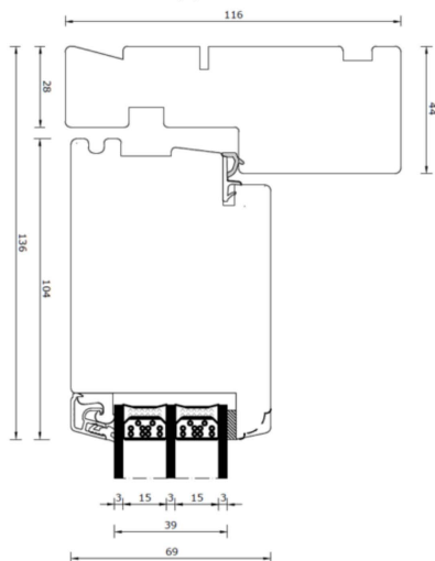
Toppkarm
