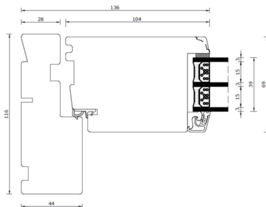
Sidokarm
