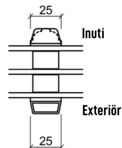
Energispröjsar
