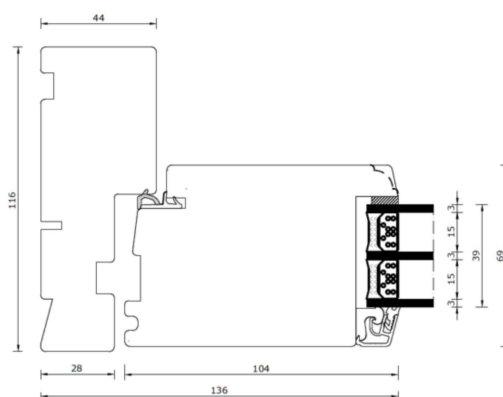
Sidokarm
