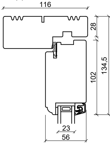
Toppkarm
