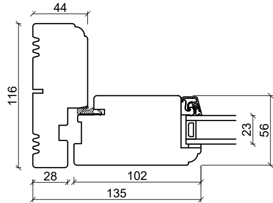
Sidokarm
