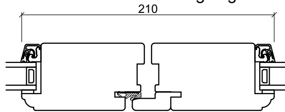
Sammenstängning
