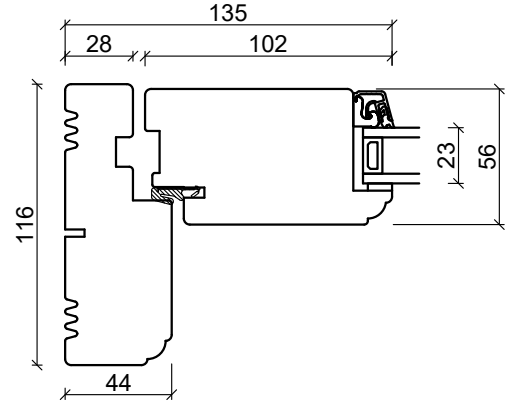
Sidokarm
