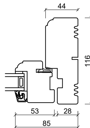
Sidokarm
