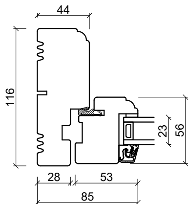
Sidokarm
