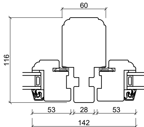
Mittpost, lodrätt
