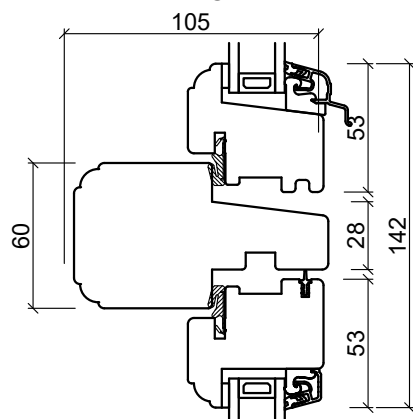
Tvärpost, vågrätt
