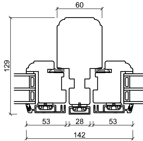
Mittpost, lodrätt
