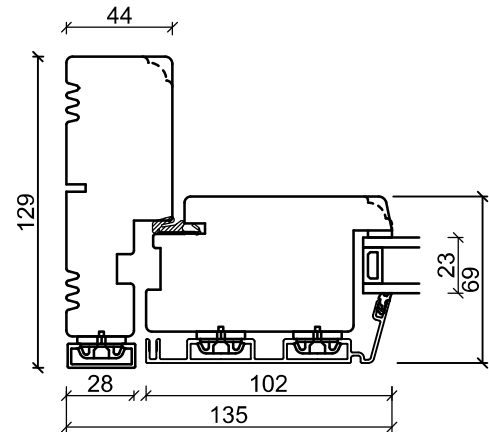
Sidokarm
