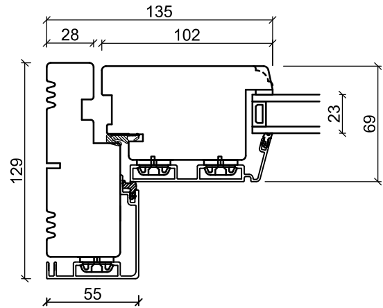
Sidokarm
