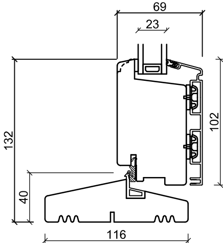
Hårdträ Bottenkarm
