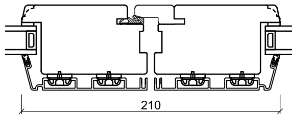
Sammenstängning
