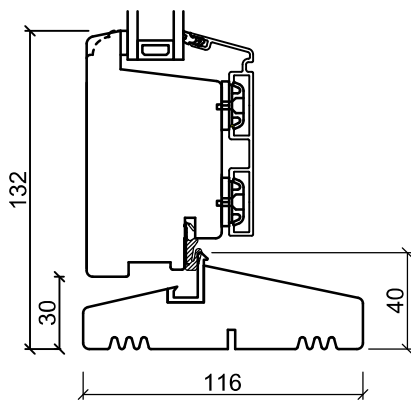
Hårdträ Bottenkarm
