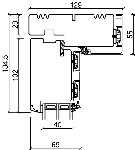
Toppkarm
