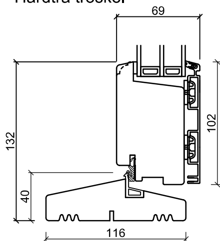
Hårdträ tröskel
