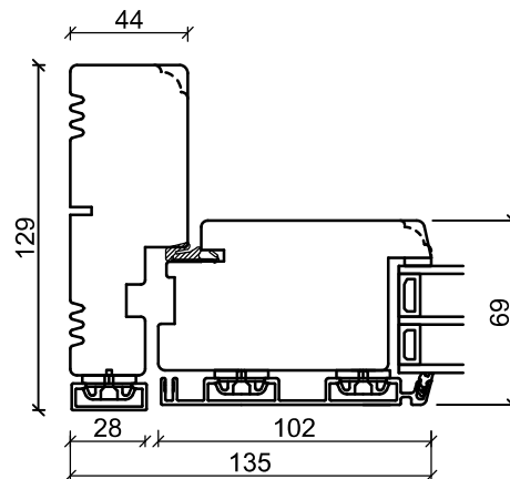
Sidokarm
