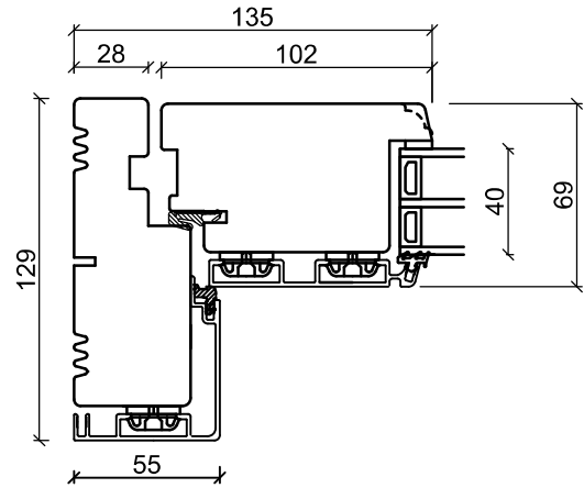
Sidokarm
