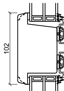
Spännstycke
