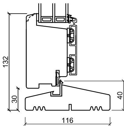
Hårdträ Bottenkarm
