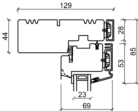
Toppkarm
