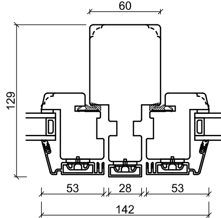
Mittpost, lodrätt
