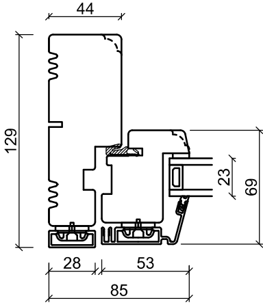
Sidokarm
