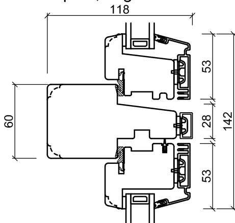
Tvärpost, vågrätt
