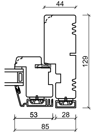
Sidokarm
