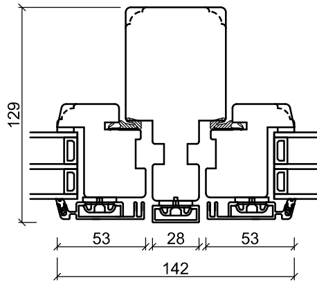
Mittpost, lodrätt
