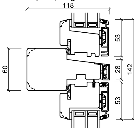
Tvärpost, vågrätt
