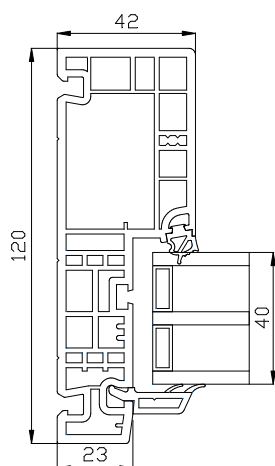
Sidokarm
