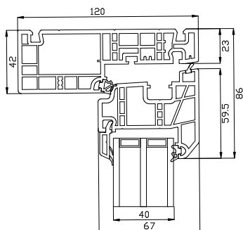
Toppkarm
