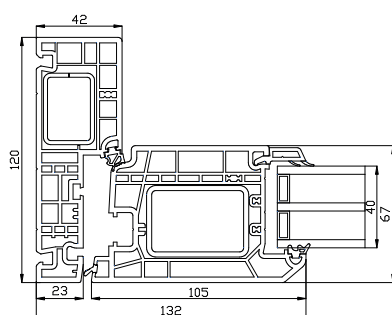
Sidokarm
