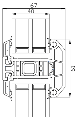
Spännstykke
