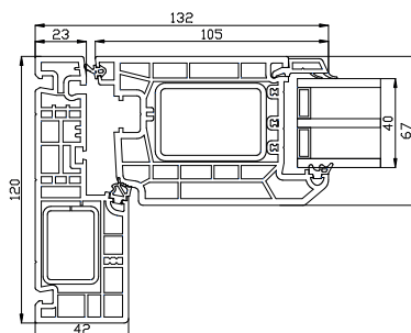
Sidokarm
