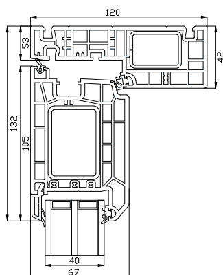
Toppkarm
