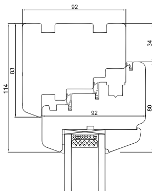
Toppkarm
