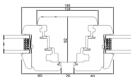
Tvärpost
