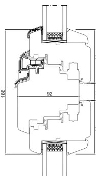
Tvärpost
