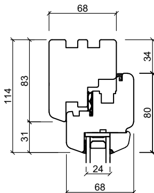
Tvärpost
