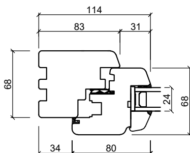
Sidokarm
