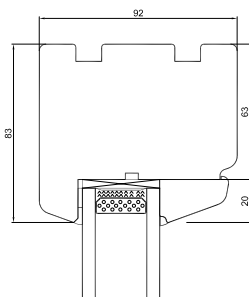
Toppkarm
