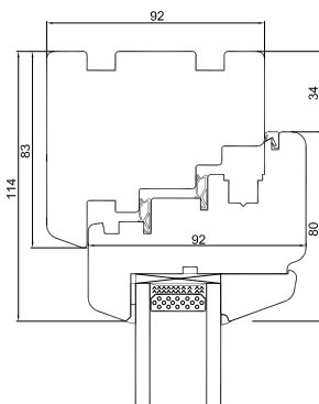
Tvärpost
