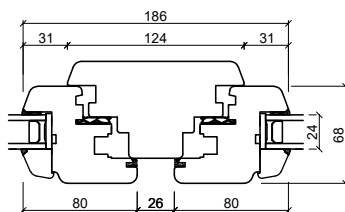
Tvärpost
