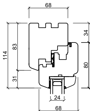
Toppkarm
