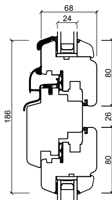
Tvärpost
