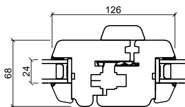
Sammanstängning
