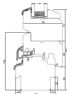
Hårdträ bottenkarm
