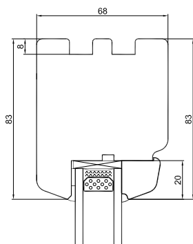
Toppkarm
