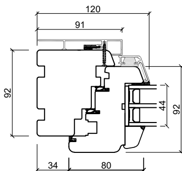
Hårdträ bottenkarm
