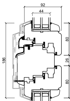
Tvärpost - vandret
