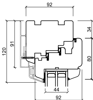
Toppkarm
