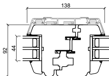
Sammanstängning
