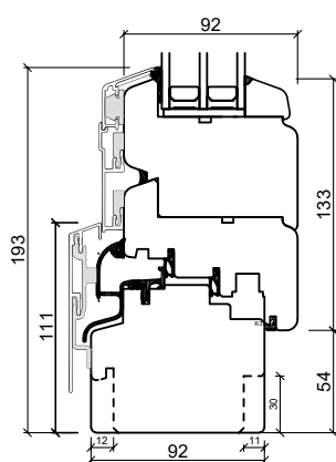
Hårdträ bottenkarm
