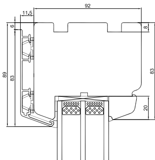
Toppkarm
