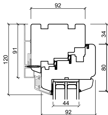
Sammanstängning
