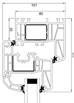
Sidokarm
