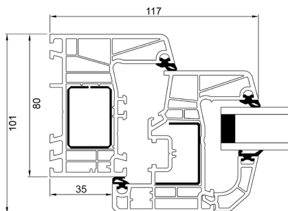
Sidokarm
