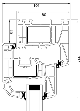
Toppkarm
