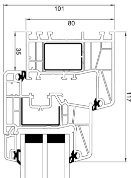
Toppkarm
