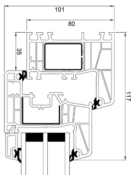
Sidokarm
