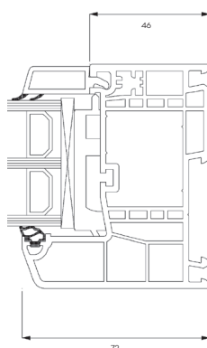
Sidokarm
