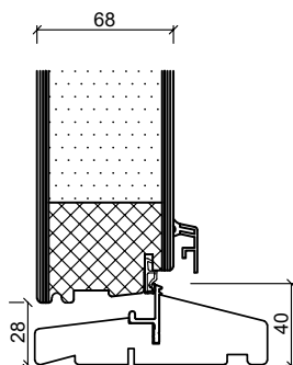
Hårdträ bottenkarm
