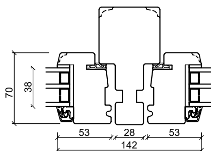
Mittpost, lodrätt
