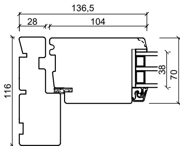
Sidokarm
