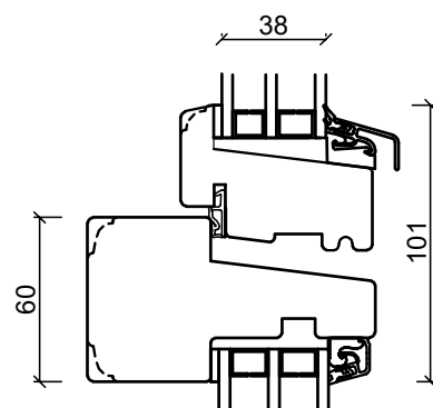
Tvärpost
