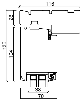
Lodret Spännstykke
