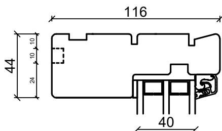
Toppkarm
