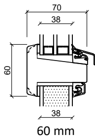
Vandret Spännstykke
