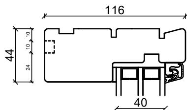
Toppkarm
