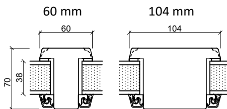
Lodret Spännstykke
