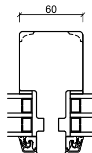
Mittpost, lodrätt
