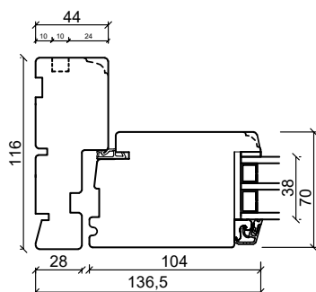
Sidokarm
