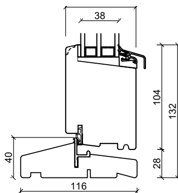
Hårdträ bottenkarm
