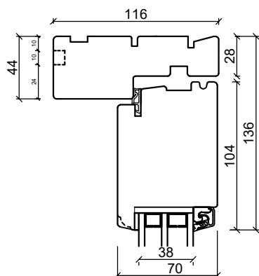
Toppkarm
