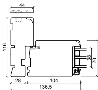
Sidokarm
