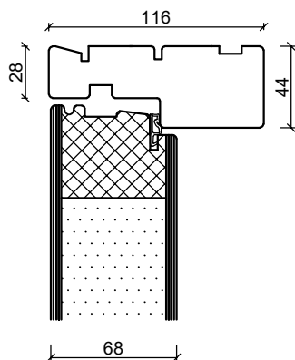
Sidokarm
