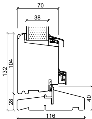
Hårdträ bottenkarm
