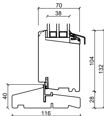
Hårdträ bottenkarm
