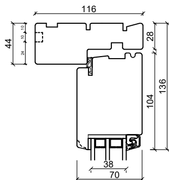
Toppkarm
