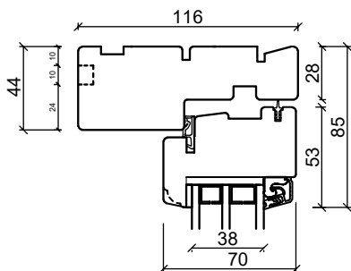
Toppkarm
