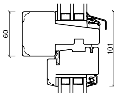
Tvärpost
