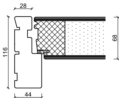
Sidokarm
