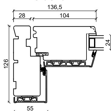
Lodret Spännstykke
