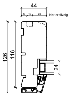
Sidokarm
