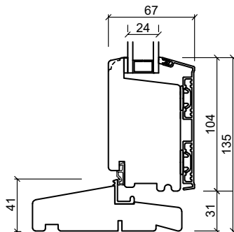
Hårdträ bottenkarm
