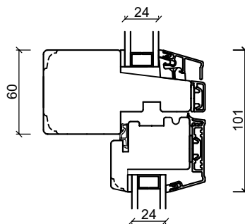
Tvärpost
