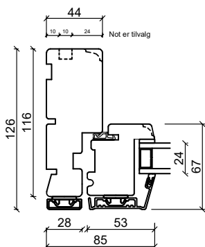
Sidokarm
