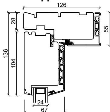
Vandret Spännstykke
