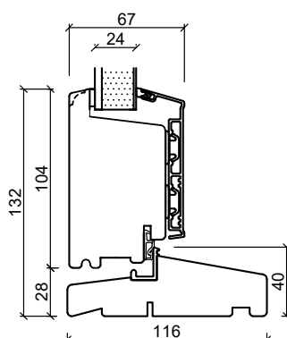
Hårdträ bottenkarm
