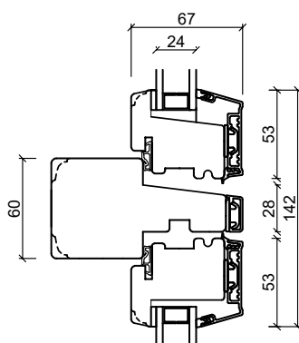
Tvärpost
