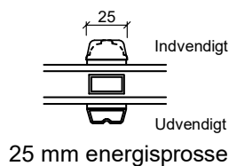
Energispröjs
