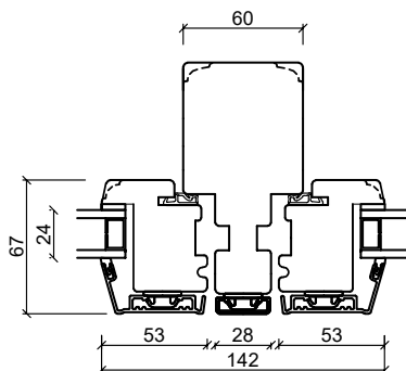
Mittpost, lodrätt
