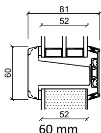
Vandret Spännstykke
