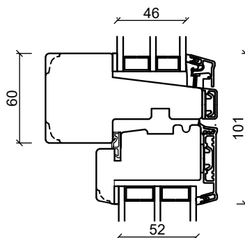
Tvärpost
