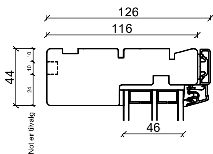
Sidokarm
