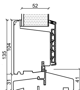
Hårdträ bottenkarm
