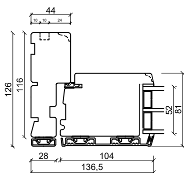
Sidokarm
