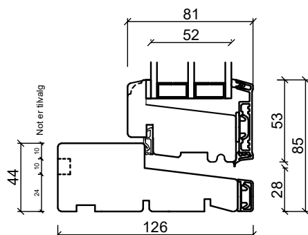
Sidokarm
