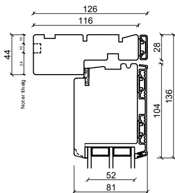
Toppkarm
