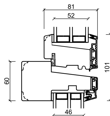
Tvärpost
