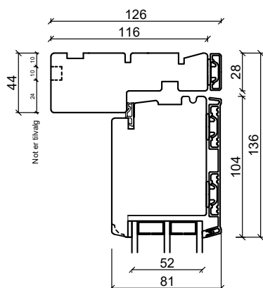
Toppkarm
