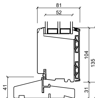
Hårdträ bottenkarm
