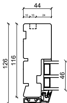
Sidokarm
