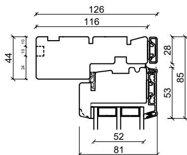
Toppkarm
