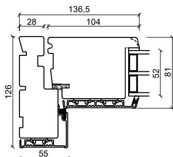
Sidokarm
