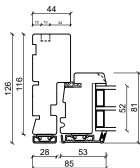
Sidokarm
