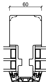
Mittpost, lodrätt
