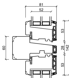
Tvärpost
