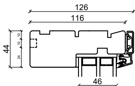
Toppkarm
