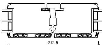
Sammanstängning
