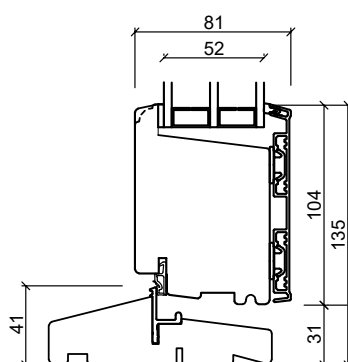
Hårdträ bottenkarm
