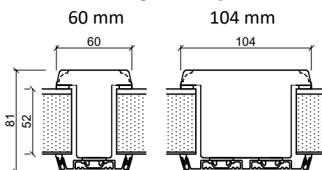
Lodret Spännstykke
